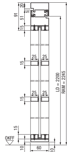
Vertikalschnitt 1-flügelige Stahl-Lofttür
