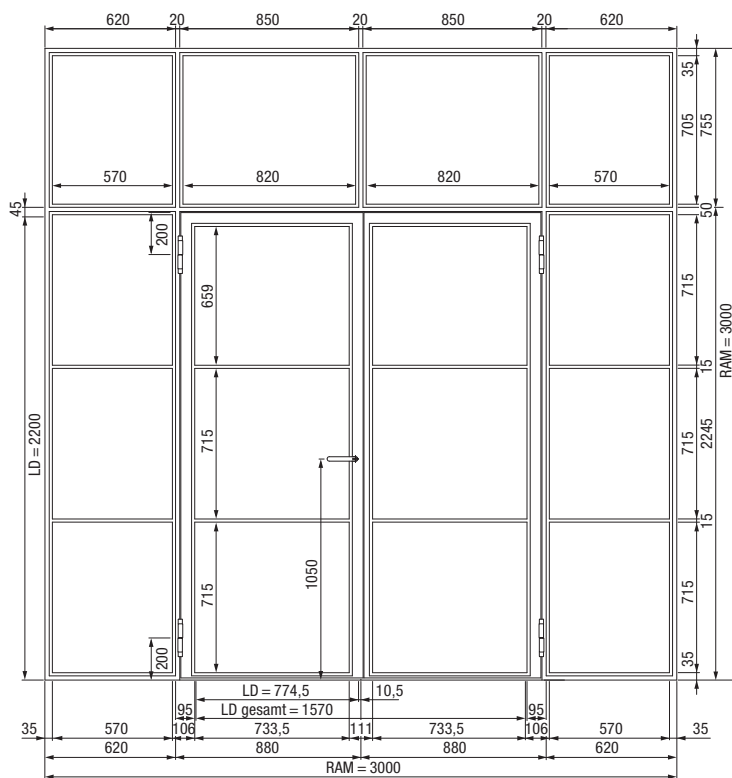
2-flüglige Stahl-Lofttür mit Seitenteilen und Oberlicht
