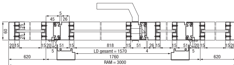
Horizontalschnitt 2-flüglige Stahl-Lofttür mit Seitenteilen
