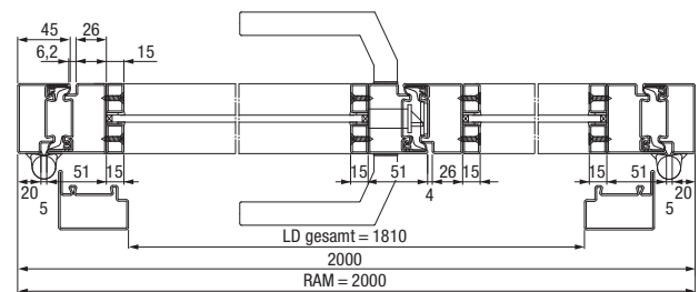
Horizontalschnitt 2-flügelige Stahl-Lofttür
