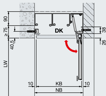
Földépcsőajtó a szemöldökhöz Teleszkópos tolókapu függőleges metszete
