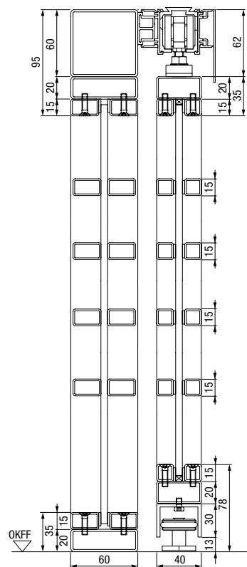
Вертикален разрез на двукрила стоманена врата с лофт дизайн със странична част
