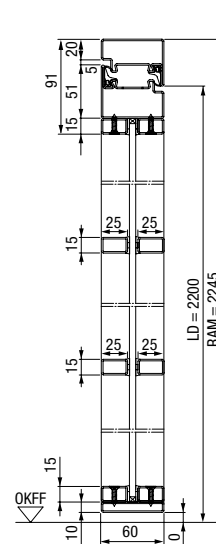
Вертикален разрез на еднокрила стоманена врата с лофт дизайн
