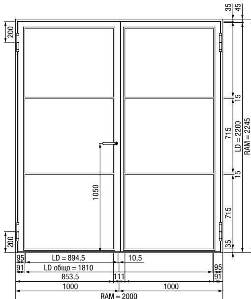
двукрила стоманена врата с лофт дизайн
