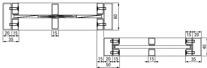
Хоризонтален разрез на двукрила стоманена врата с лофт дизайн със странична част
