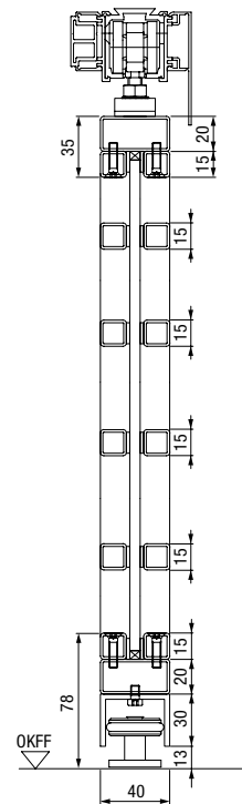
Вертикален разрез на двукрила стоманена врата с лофт дизайн
