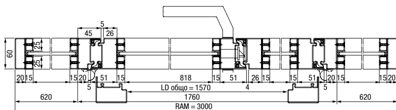
Хоризонтален разрез на двукрила стоманена врата с лофт дизайн със странични части
