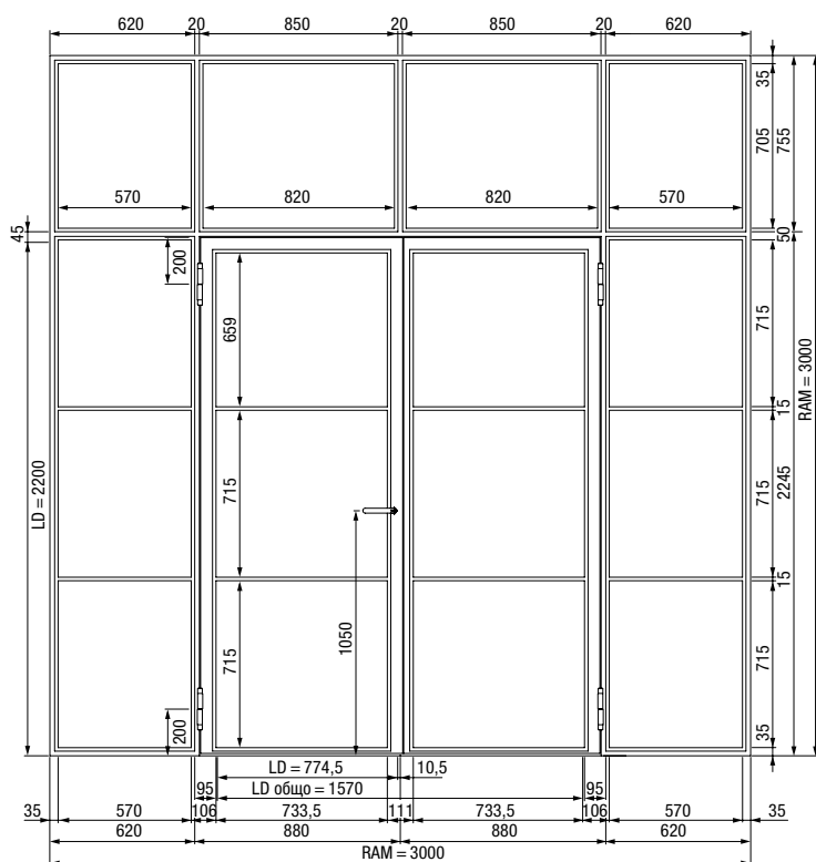
двукрила стоманена врата с лофт дизайн със странични части и оберлихт
