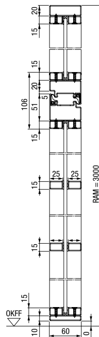
Вертикален разрез на еднокрила стоманена врата с лофт дизайн с оберлихт
