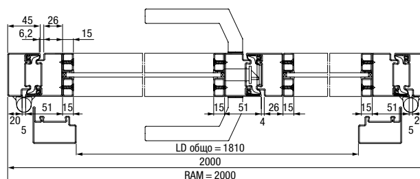
Хоризонтален разрез на двукрила стоманена врата с лофт дизайн
