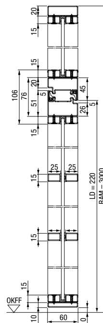
Вертикален разрез на двукрила стоманена врата с лофт дизайн с оберлихт
