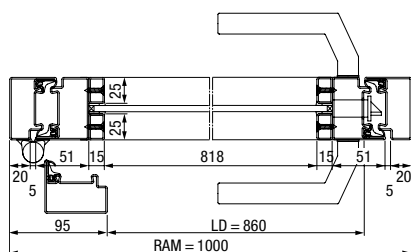
Хоризонтален разрез на еднокрила стоманена врата с лофт дизайн
