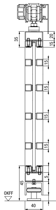
Przekrój pionowy
