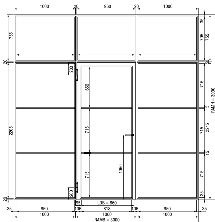
1-skrzydłowe drzwi rozwerne z naświetlami bocznymi i naświetlem górnym
