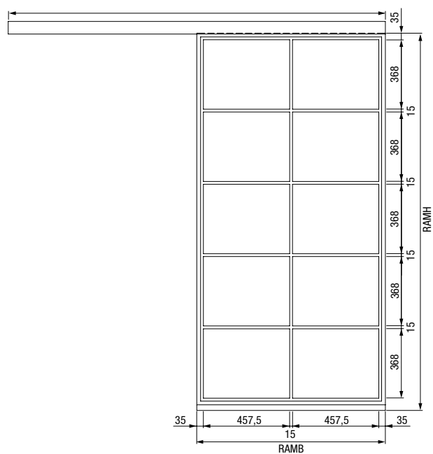
1-skrzydłowe drzwi przesuwne
