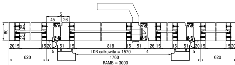
Przekrój poziomy
