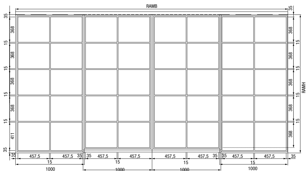
2-skrzydłowe drzwi przesuwne z elementami bocznymi
