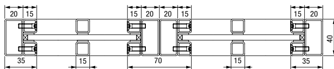
Przekrój poziomy
