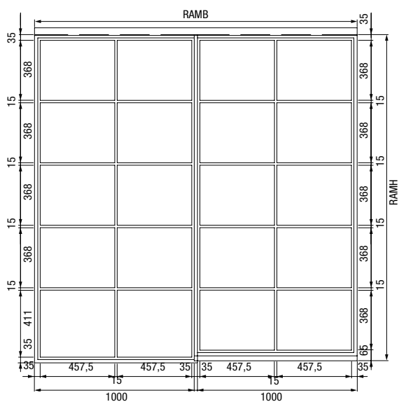
1-skrzydłowe drzwi przesuwne z naświetlem bocznym
