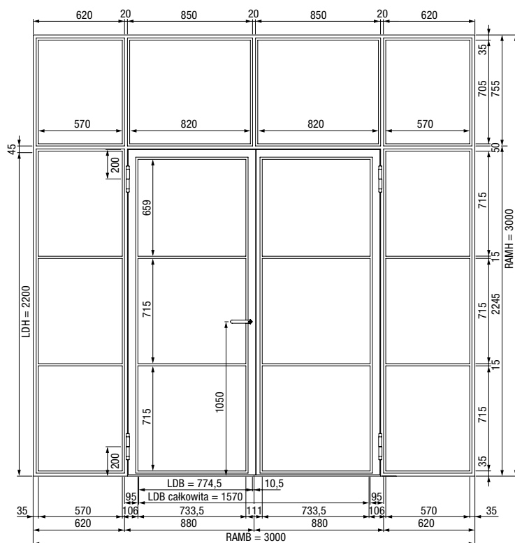
2-skrzydłowe drzwi rozwierne z naświetlami bocznymi i naświetlem górnym
