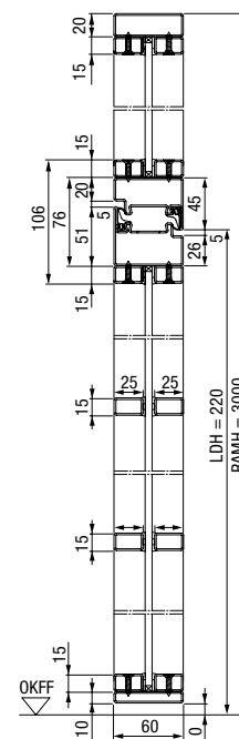
Przekrój pionowy
