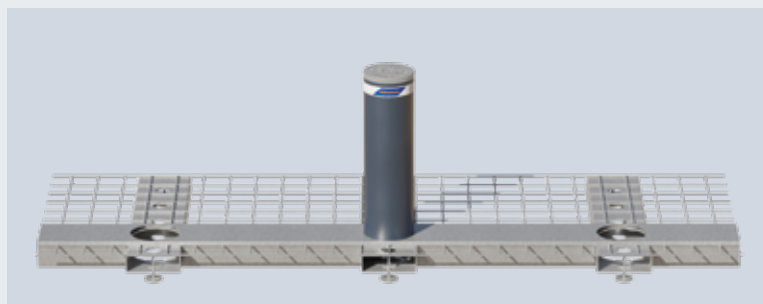
Standard aljzati rögzítés 1 fix hengerrel (elrendezés a forgalmi irány közepén), opcióban jobbos vagy balos kivitelben
