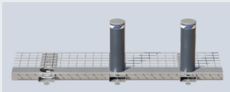
Standard aljzati rögzítés 2 fix hengerrel (elrendezés a forgalmi irány közepén / jobbos), közepén / balos elrendezés is lehetséges
