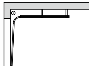
Направляющая N Стандартная направляющая
