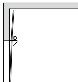
Направляющая VU с низко расположенным пружинным валом
