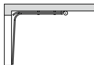
Tipo de guías L Guías con muelle trasero
