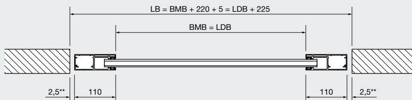
Przekrój poziomy Montaż przed lub za otworem (przykład z prowadnicą FS 110 x 100*)
