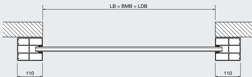
Przekrój poziomy Montaż przed lub za otworem (przykład z prowadnicą FS 110 x 100*)
