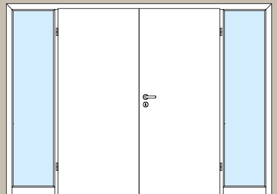
2-vleugelig, 2 zijdelen
