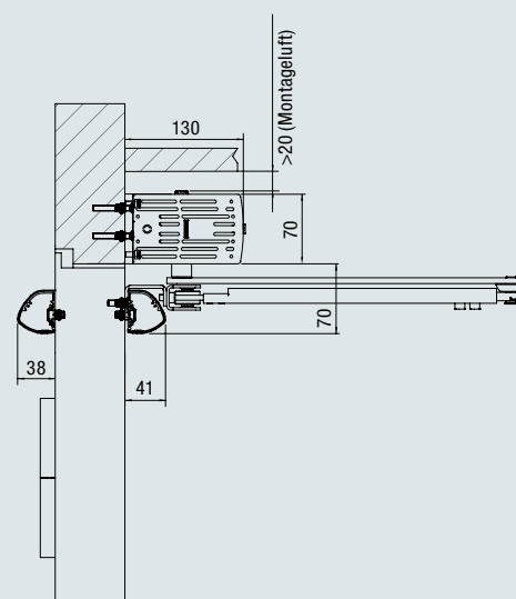
Montage auf Bandgegenseite, drückend
