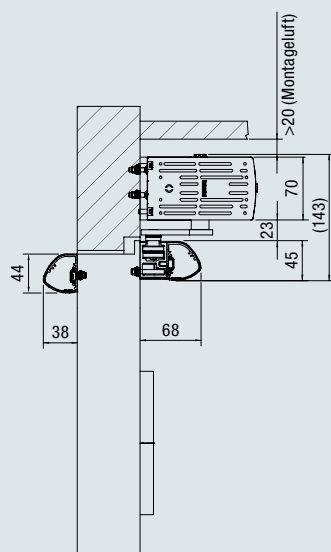
Montage auf Bandseite, ziehend
