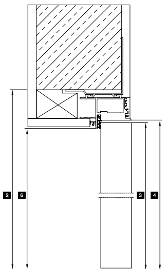
Vertikalni presek krila vrata bez falca, koje se otvara unazad
