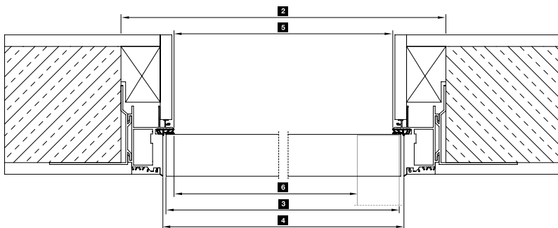
Horizontalni presek krila vrata bez falca
