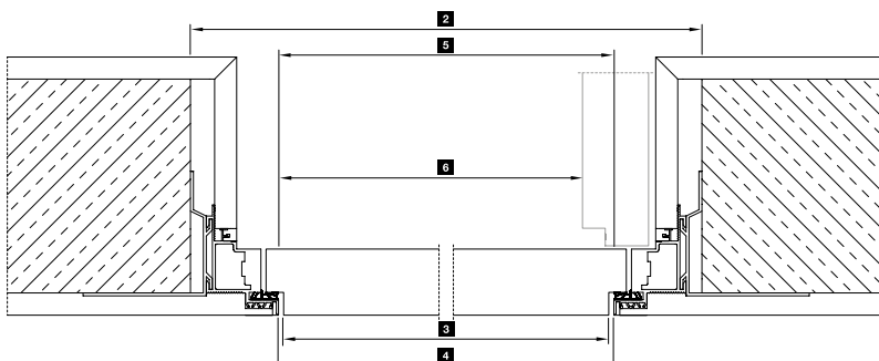
Horizontalni presek krila vrata bez falca, koje se otvara unazad
