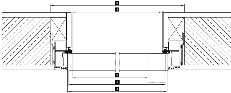
Horizontalschnitt mit stumpfem Türblatt
