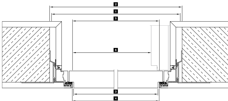
Przekrój poziomy z rewersyjnym skrzydłem drzwiowym
