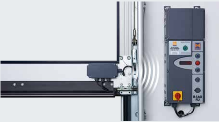
Trådløs overføringsenhet Ekstrautstyr for signaloverføring fra portbladet via Bluetooth til styringen – i stedet for en spiralledning. Strømforsyningen skjer via et kraftig batteri. Komponenter som kan tilkobles: Optosensorer LE (lavenergi), underliggende fotocelle VL 1/2-LE, 8k2-list, wireslakk-bryter, gangdørkontakt, kontakt for nattlås
