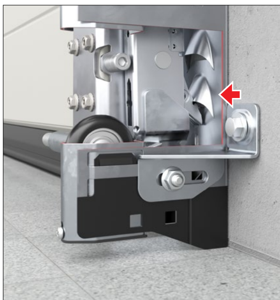
Zatrzask ryglujący w kształcie haka blokuje się automatycznie przy próbie podważenia bramy.
