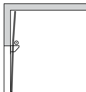
Prowadzenie VU z obniżonym wałem sprężyny skrętnej
