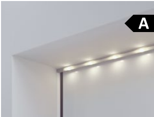
Listwa świetlna LED do bram neutralne białe światło, indywidualny, skracany system wtykowy, montaż pod nadprożem (na ilustracji) lub na dolnej krawędzi płyty bramy
