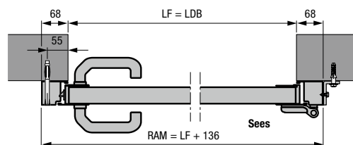
Alumiiniumist karplengiga kõrvaluks, profiilitüüp 2 Paigaldus ava taha
