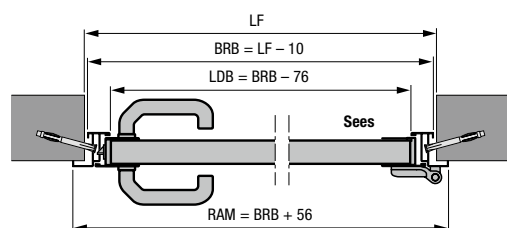
Alumiiniumist nurklengiga kõrvaluks, profiilitüüp 2 Seespoolne paigaldusruum
