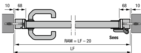
Alumiiniumist karplengiga kõrvaluks, profiilitüüp 2 Paigaldus ava sisse
