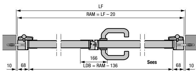
Kahe lehega alumiiniumist karplengiga kõrvaluks, profiilitüüp 2 Paigaldus ava sisse
