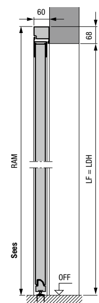
Alumiiniumist karplengiga kõrvaluks, profiilitüüp 2 Paigaldus ava taha
