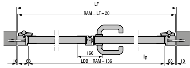
Alüminyum blok kasalı çift kanatlı yan kapı profil tipi 2 Açıklıkta montaj
