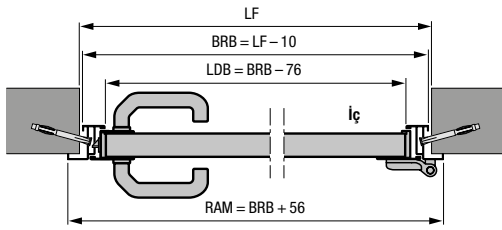
Alüminyum köşe kasalı yan kapı profil tipi 1 veya 2 İç montaj
