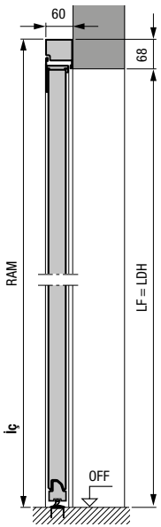
Alüminyum blok kasalı yan kapı profil tipi 2 Açıklığın arkasına montaj
