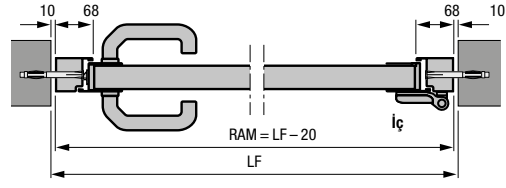
Alüminyum blok kasalı yan kapı profil tipi 2 Açıklıkta montaj
