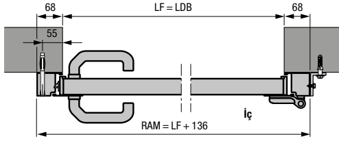
Alüminyum blok kasalı yan kapı profil tipi 1 Açıklığın arkasına montaj
