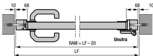
Bočna vrata sa aluminijumskim obuhvatnim štokom, tip profila 2 Ugradnja u otvoru
