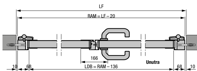
2-krilna bočna vrata sa aluminijumskim obuhvatnim štokom, tip profila 2 Ugradnja u otvoru
