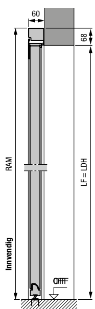
Sidedør med blokkarm av aluminium, profiltipe 2 Montering bak åpningen
