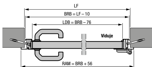
Šoninės durys su aliuminine kampine stakta, 1 arba 2 profilio tipas Vidinė atrama
