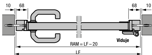
Šoninės durys su aliuminine blokine stakta, 2 profilio tipas Įstatymas angoje
