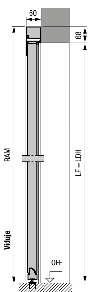
Šoninės durys su aliuminine blokine stakta, 2 profilio tipas Įstatymas už angos
