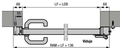
Šoninės durys su aliuminine blokine stakta, 1 profilio tipas Įstatymas už angos
