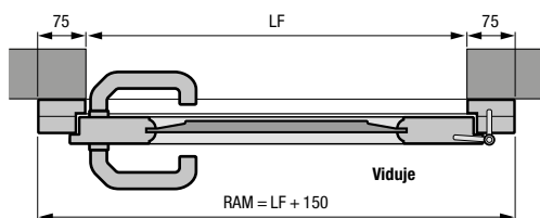
Šoninės durys iš masyvinės medienos Įstatymas už angos
