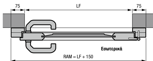
Πλαϊνή πόρτα από μασίφ ξύλο Τοποθέτηση πίσω από το άνοιγμα
