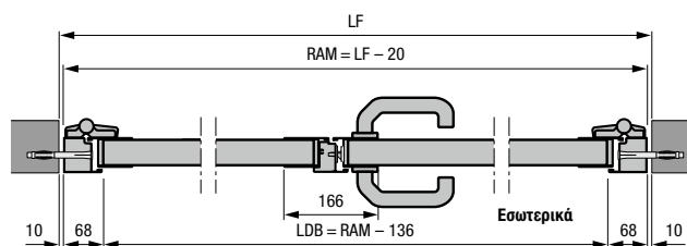
Δίφυλλη πλαϊνή πόρτα με απλή κάσα αλουμινίου προφίλ τύπου 2 Τοποθέτηση στο άνοιγμα
