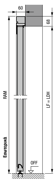
Πλαϊνή πόρτα με απλή κάσα αλουμινίου προφίλ τύπου 2 Τοποθέτηση πίσω από το άνοιγμα
