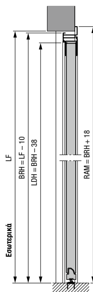
Πλαϊνή πόρτα με γωνιακή κάσα αλουμινίου προφίλ τύπου 2 Άνοιγμα προς τα έξω
