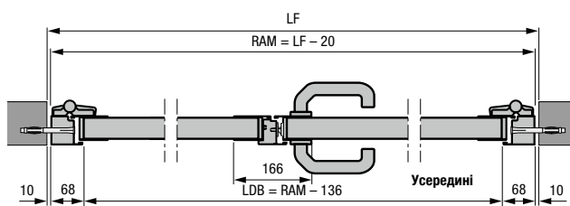
2-стулкові бічні двері з алюмінієвою блочною коробкою, тип профілю 2 Монтаж в отворі
