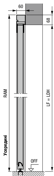
Бічні двері з алюмінієвою блочною коробкою, тип профілю 2 Монтаж за отвором
