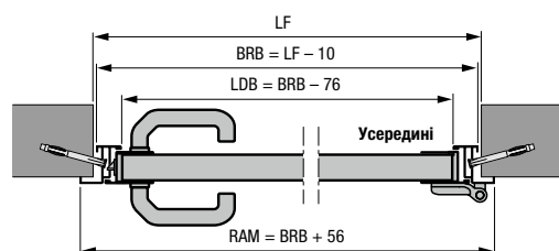
Бічні двері з алюмінієвою кутовою коробкою, тип профілю 2 Внутрішній упор
