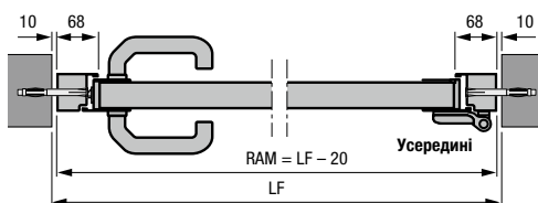
Бічні двері з алюмінієвою блочною коробкою, тип профілю 2 Монтаж в отворі
