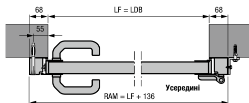
Бічні двері з алюмінієвою блочною коробкою, тип профілю 2 Монтаж за отвором
