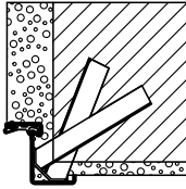
Ankrajlı montaj
