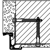
Vidalı montaj
