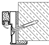
Çapraz sabitleme (Sıvasız tuğla duvar / beton)
