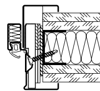
Çapraz sabitleme (Gazbeton)
