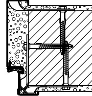
Köşe ve ek kasa Vidalı montaj
