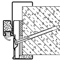
Çapraz sabitleme 2 cidarlı tam kasa olarak ilave kasa Vario B53 ile (Gazbeton)
