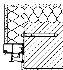
Štok u obliku bloka Montaža sa ankerima
