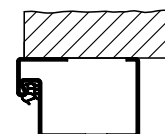
Štok u vidu bloka za montažu na zid (profil 006) (testirano na strani suprotno od šarki)
