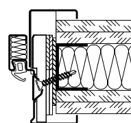
Dijagonalno pričvršćivanje (porobeton)
