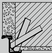
Τοποθέτηση με αγκύρια τοιχοποιίας
