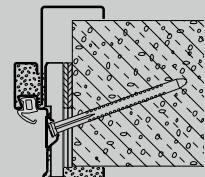
Διαγώνια στερέωση με πρόσθετο κούφωμα Vario B53 ως κάσα σχήματος U 2 κελύφων (ελαφρομπετόν)
