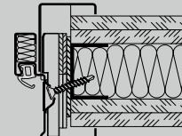
Διαγώνια στερέωση (ελαφρομπετόν)
