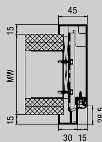
Προφίλ 21180, με πλατύ καβαλίκι
