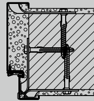
Γωνιακή και συμπληρωματική κάσα Τοποθέτηση με αγκύρια με βύσματα
