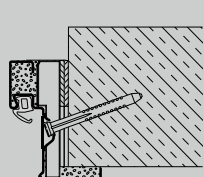
Διαγώνια στερέωση (Τοιχοποιία/μπετόν)
