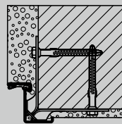
Τοποθέτηση με αγκύρια με βύσματα
