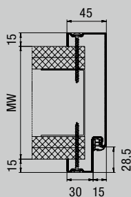
Προφίλ 21120, στερέωση με αντικριστές βίδες
