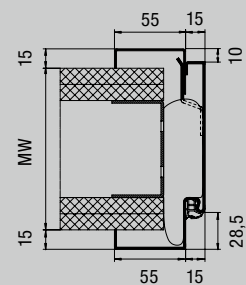
Προφίλ 31103, με πλατύ καβαλίκι
