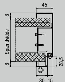
Profil 21120
