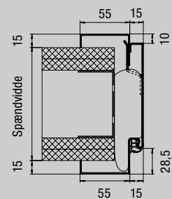
Profil 31103, falset
