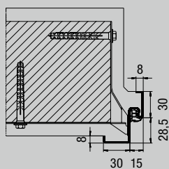
Profil 11100
