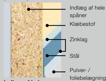
Indlæg af hele spåner (ekstraudstyr) giver forbedret lydisolering
