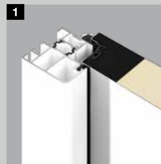
Sikkerhedsdøren KSI Thermo46 imponerer med et 46 mm tykt dørblad og en meget god isoleringsværdi på ned til 1,1 \text{ W}/(\text{m}^2 \cdot \text{K}) .
