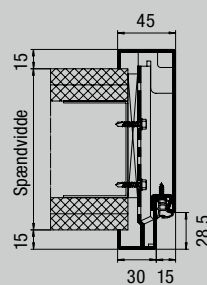
Profil 21180, falset
