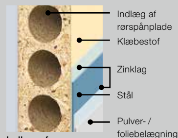
Indlæg af rørspånplade (standard)
