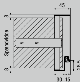
Profil 21101
