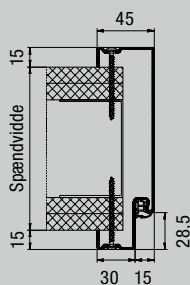
Profil 21120, spejl-skruemontering
