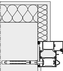
Huisserie à rupture de pont thermique Montage rapide
