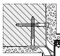
Pose avec pattes d'ancrage à cheviller
