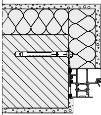
Huisserie à rupture de pont thermique Montage par pattes d'ancrage
