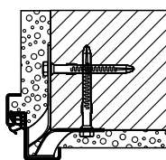
Montering med dyveforankring
