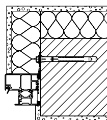
Standardkarm Montering med forankring
