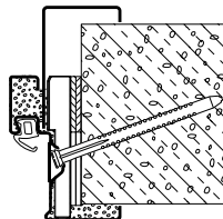
Diagonalfastgørelse med supplerende karm Vario B53 som yderkarm i 2 dele (gasbeton)
