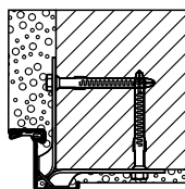
Montering med dyvelforankring
