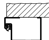
Standardkarm til montering på væggen (profil 006) (kontrolleret på den modsatte side af hængslet)
