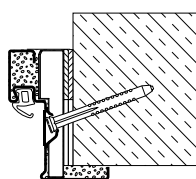
Diagonalfastgørelse (synligt murværk / beton)
