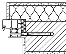
Standardkarm Montering i murværk Montering med borehuller
