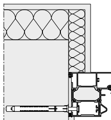
Ościeżnica blokowa Montaż przelotowy
