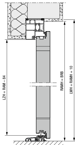
Przekrój pionowy
