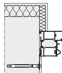
Ościeżnica blokowa do montażu w otworze (profil 21101)
