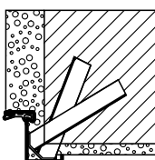
Beépítés horgonyos rögzítőelemmel
