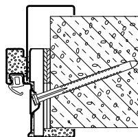
Átlós rögzítés Vario B53 kiegészítőkkal 2-részes befoglalótként (Gázbeton)
