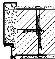
Sarok- és kiegészítőtok Beépítés tiplis rögzítőelemmel
