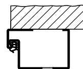
Karpleng paigaldamiseks seina peale (profiil 006) (hingede vastaspool kontrollitud)
