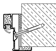
Diagonaalkinnitus (viimistlust mittevajav müüritis / betoon)
