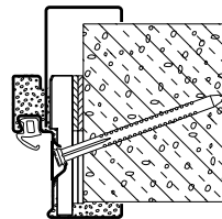
Diagonaalkinnitus laienduslengidega Vario B53 kaheosalise põski ümbritseva lengina (gaasbetoon)
