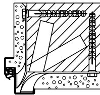
Nurkleng Paigaldus müüritisse Lengitüübel
