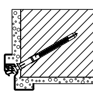
Eri-nurkleng Paigaldatakse tüüblitega läbi lengi
