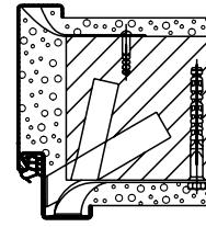
Põski ümbritsev leng Paigaldus müüritisse Lengitüübel
