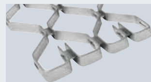
HG-V, aluminijum (ojačan); HG-S, čelik 12000 × 8000 mm
