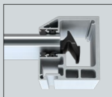
Haki przeciwwiatrowe W4 (brama rolowana)
