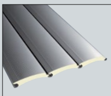
Decotherm S, stal szerokość bramy maks.: 5000 mm wysokość bramy maks.: 2400 mm
