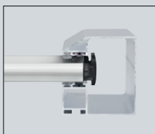
Haki przeciwwiatrowe z tworzywa sztucznego, dostępne standardowo (brama rolowana)
