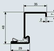
Huissierie d'angle spéciale pour montage dans maçonnerie et béton
