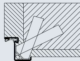
Huissierie d'angle spéciale avec pattes de scellement
