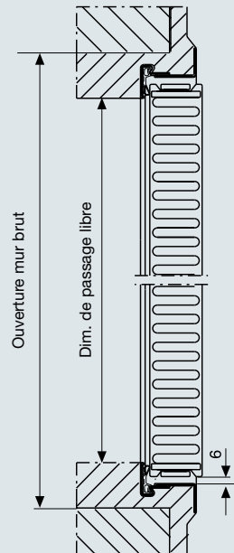
Représentation avec cornière interchangeable (avec seuil)
