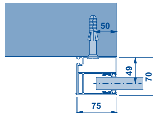
Sans chambre de ressorts
