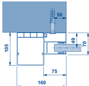
Avec chambre de ressorts et AFK
